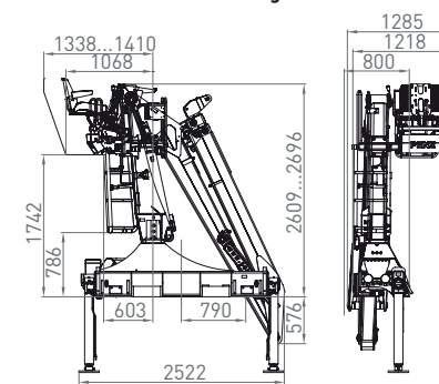
Seitensitz 02 universal rechts & links Side seat 02 universal right & left
