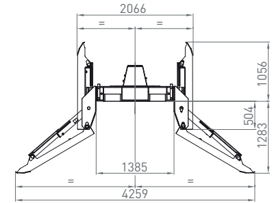
Klappabstützung Folding support
