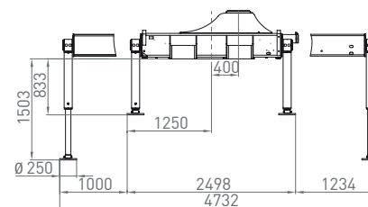
Socket seitenverkehrt Crane base Inverted
