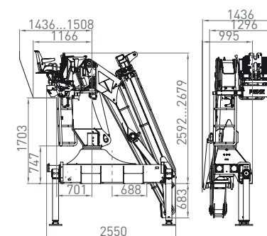
Seitensitz 02 universal rechts & links side seat 02 universal right & left
