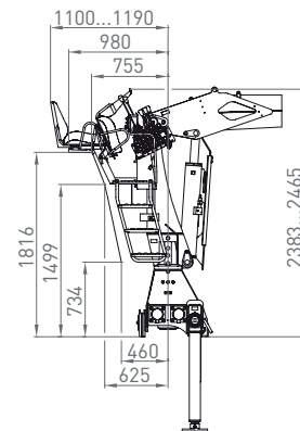
Rücksitz 01 Back seat 01
