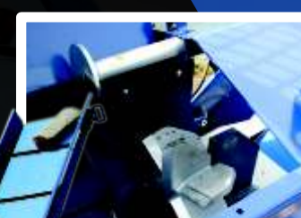
Omezovač délky je seřiditelný od 25 do 50 cm po 5 cm
