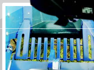
Mezi štípacím nožem a dopravníkem je zabudována mříž pro zachycování pilin.
